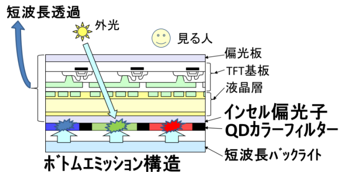
図1：インセル偏光子とQDカラーフィルターを使用したボトムエミッション型ディスプレイの構造
